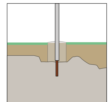
Förankring i berg/mark: Stolpen förankras i berg med stolpdubb och toppgjuts.
