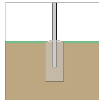
Direktgjutning: Stolpen gjuts med betong direkt i marken.
