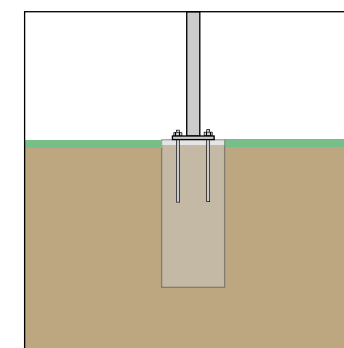
Fotplatta: Stolpen monteras med gångstänger/expanderbult på plint/platta.
