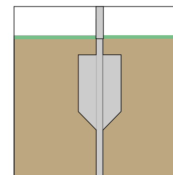
Markrör med vinge: Stolpen monteras på nerdrivet markrör med vinge.
